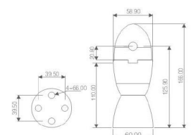
Adjustable Support Leg : Опора регулируемая Width Selection is available (оптимальная ширина наполнения 12-18мм) Height Selection is available (оптимальная высота наполнения 110-130мм)
