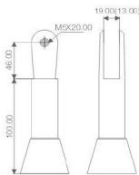
Adjustable Support Leg | Опора регулируемая Width Selection is available (определ. шир. 12-18 мм) Height Selection is available (оптимальная высота наполнения (Optimum height: 95-130mm))
