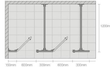
Horizontal Drawing Горизонтальный чертёж
