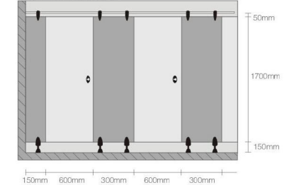
Front Vertical Drawing Вертикальный чертёж
