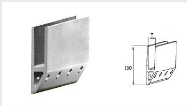
JRS-8634 玻璃托架 Glass bracket
