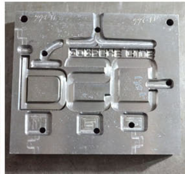
06 Zinc alloy die casting mould
